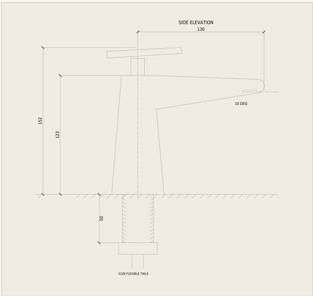
SIDE ELEVATION · SHORT BODY · 1:1 · DIMENSIONS IN MM
