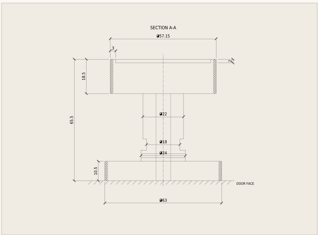
SECTION A-A · 2:1 · DIMENSIONS IN MM
