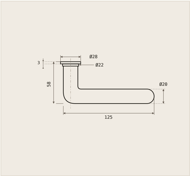
SIDE ELEVATION · 1:2 · DIMENSIONS IN MM
