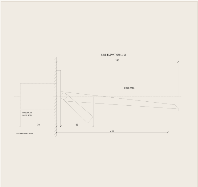
SIDE ELEVATION · 1:1 · DIMENSIONS IN MM
